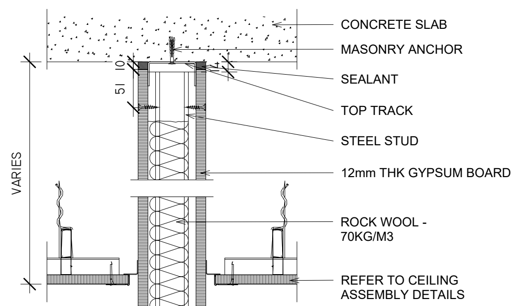
4 TYP. SOUND PROOFING 1 : 5
