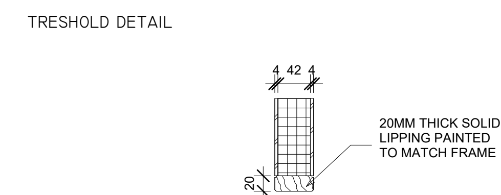
15 TYP. FLUSH WOOD DOOR DETAILS 1 : 5
