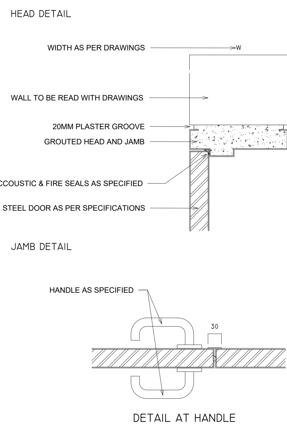
16 TYP. STEEL DOOR DETAILS 1 : 5
