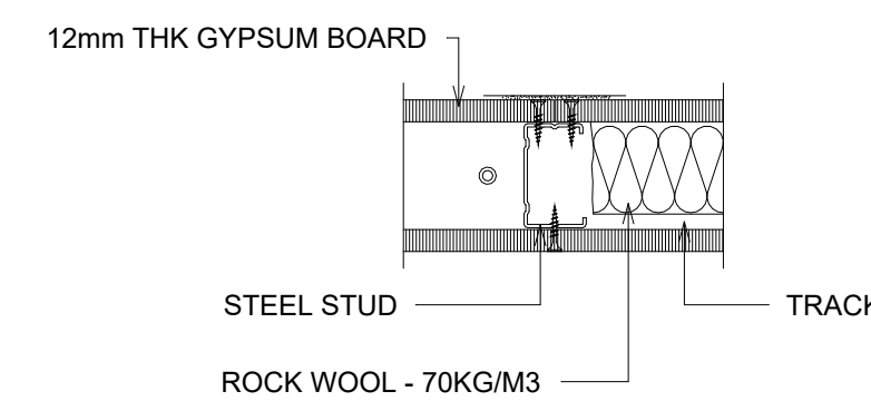
6 TYP. BUTT JOINT 1 : 5
