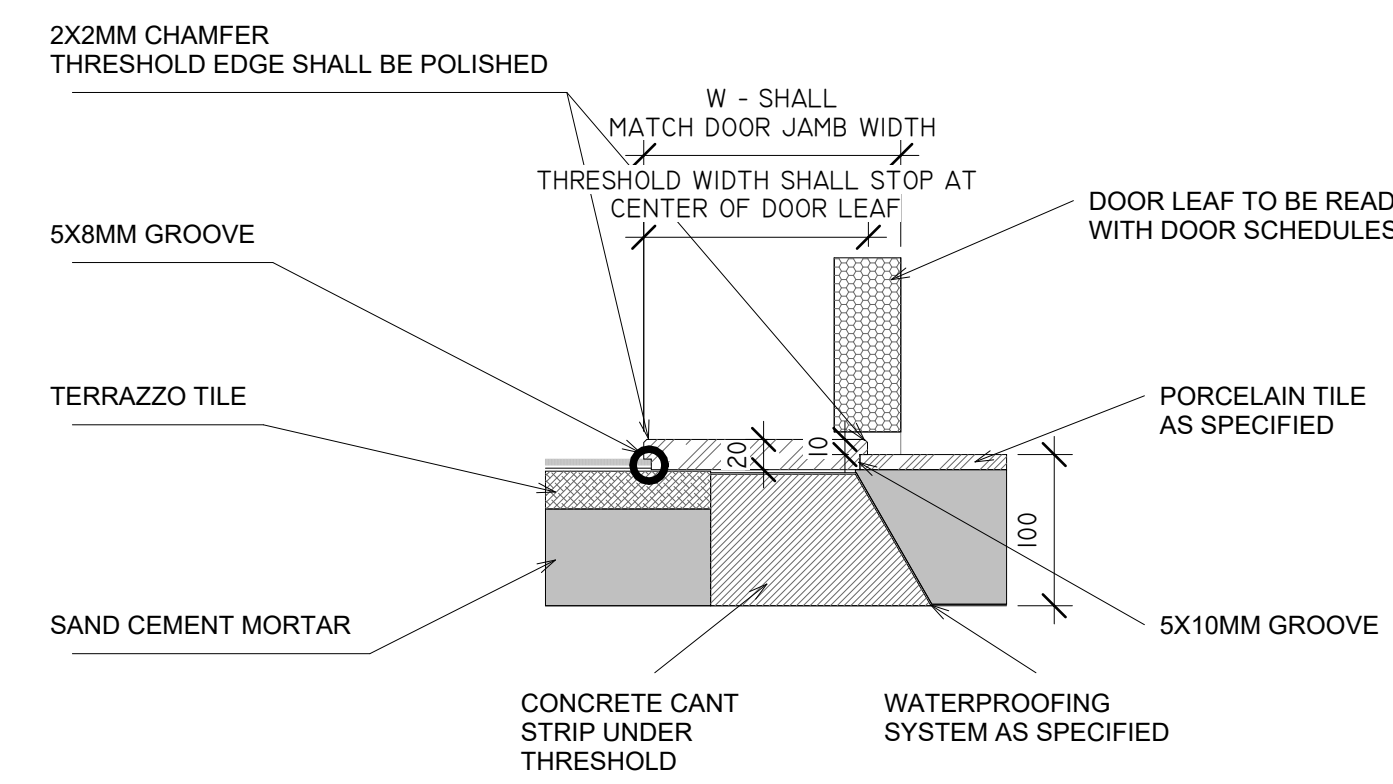
10 TYP. TOILET THRESHOLD DETAIL 1 : 5
